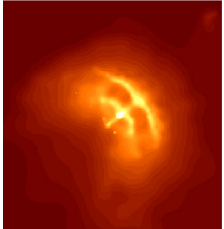
Vela Pulsar
