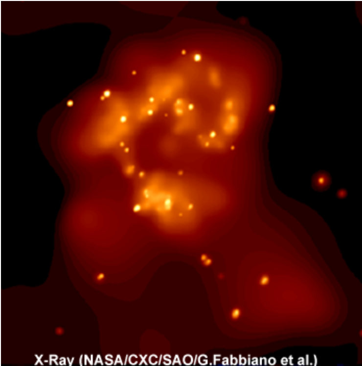
X-Ray (NASA/CXC/SAO/G.Fabbiano et al.)
