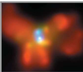
NGC 6240
